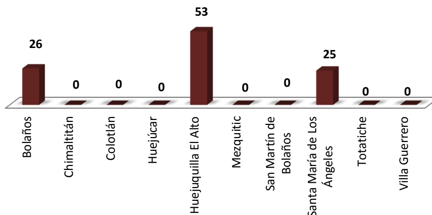
Figura 4. Aguas residuales tratadas (%) en la región Norte, 2012.
