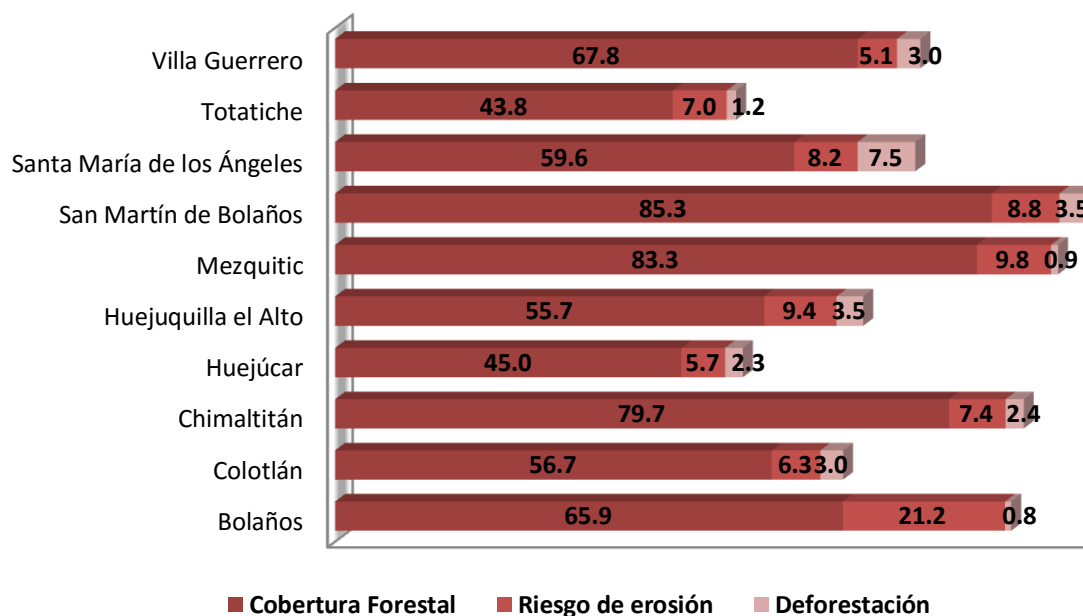
Figura 3. Cobertura forestal, riesgo de erosión y deforestación (%) en la región Norte, 2010.
